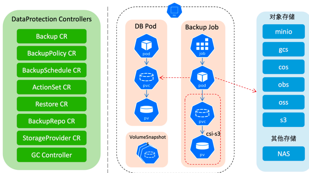
图 11. KubeBlocks Enterprise 备份中心
